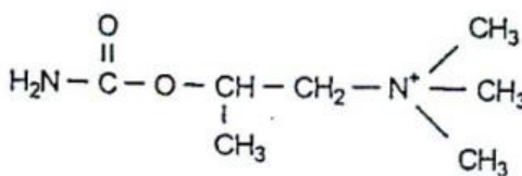
Betanechol
