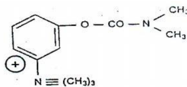
Prostigmin
