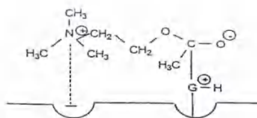
Phức hợp
