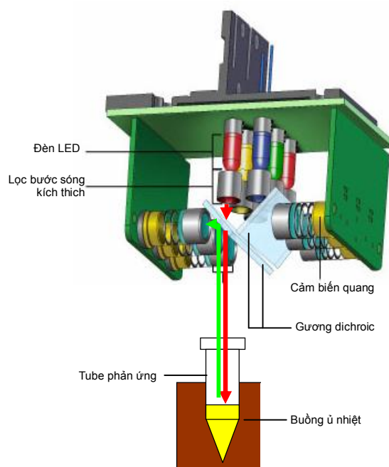
Hình 22: Hệ thống 6 đèn LED cùng với 6 cảm biến quang được gắn trên một giá và được di chuyển sát trên bể ủ nhiệt có trong thiết bị Real-time PCR của máy real-time PCR CFX 96 của Biorad
